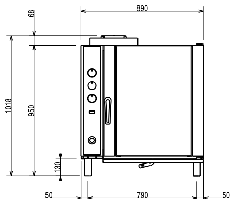
Oldalnézet
